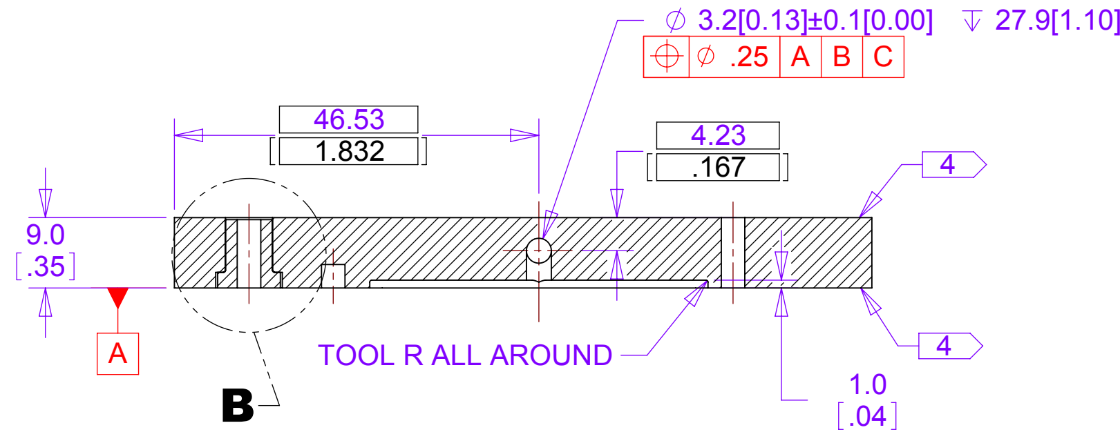
SECTION A-A
